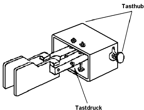
Geberjustage ETM-9C
