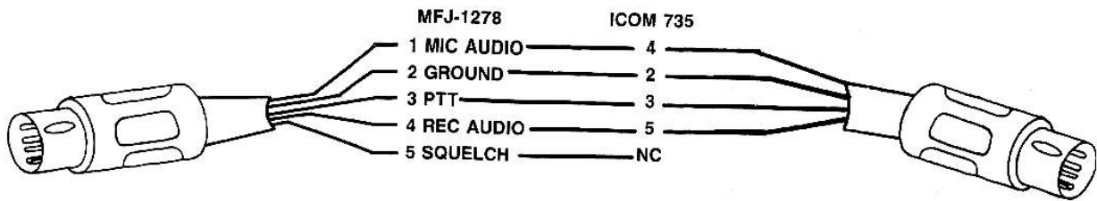
5-PIN DIN TO 1278
