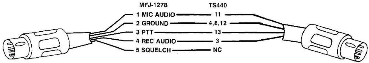
5-PIN DIN TO 1278
