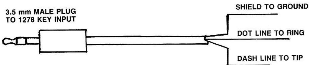
CW Key Paddle Cable
